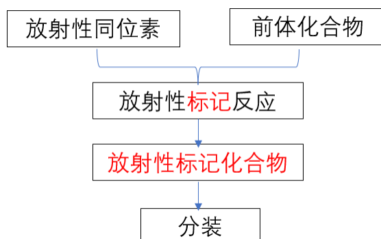
图 9-2 放射性分子探针标记工艺流程图
