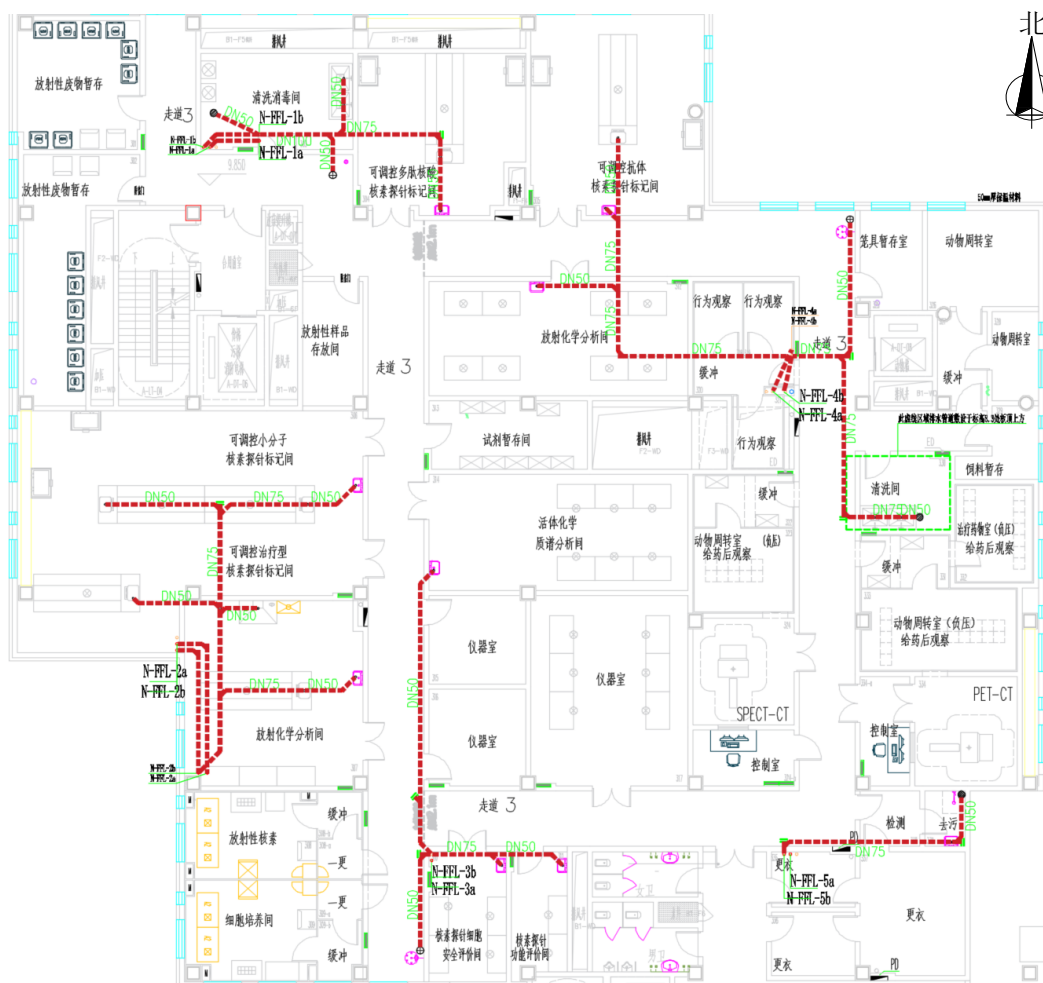
图 10-7 四层放射性废水路由图
