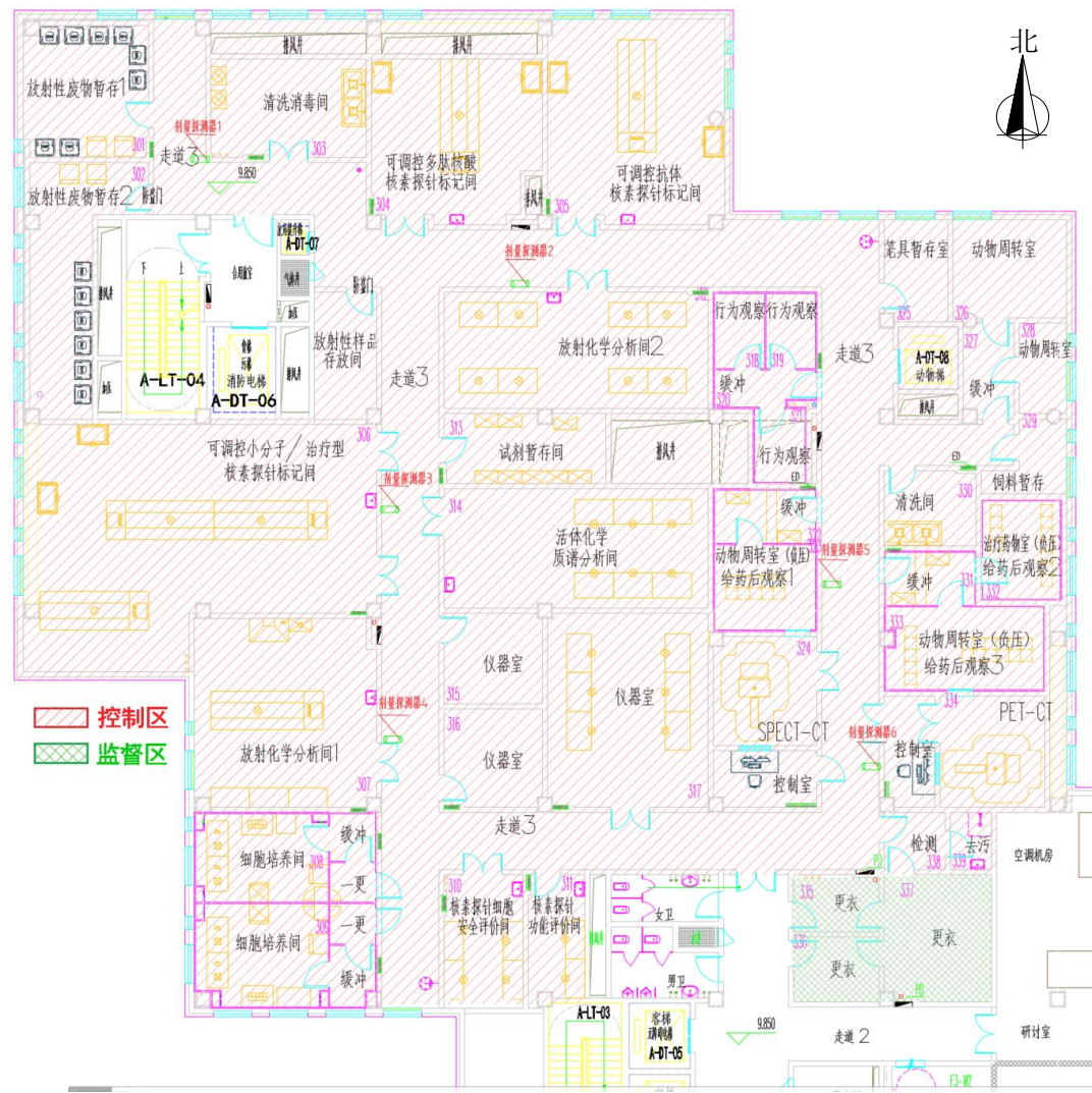
图 10-2 本项目放射性同位素实验室平面布局图
