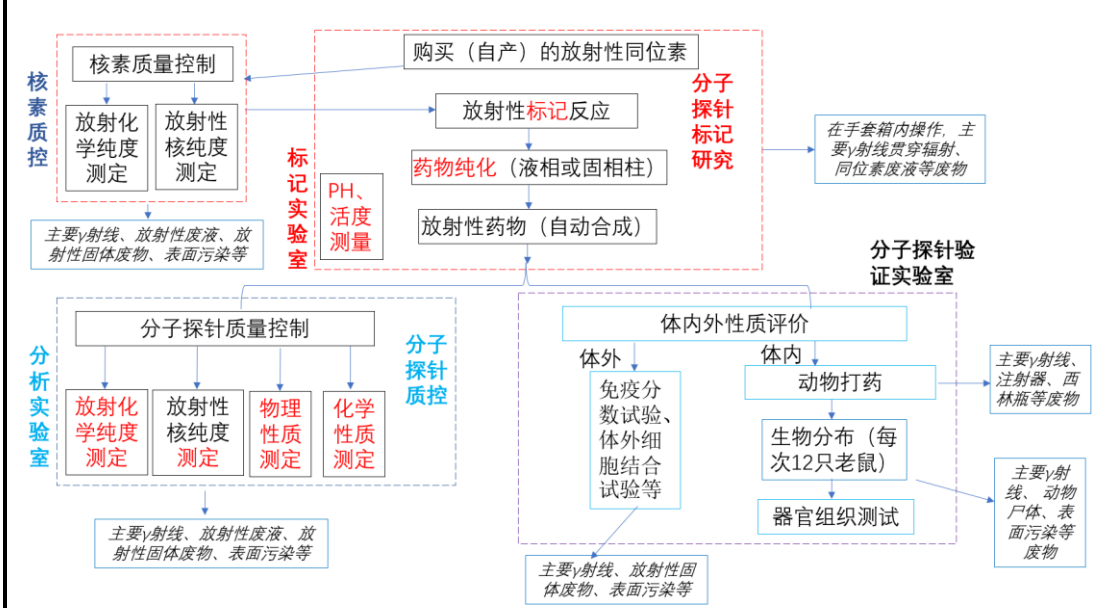
图 9-1 本项目实验工艺流程和产污环节示意图
