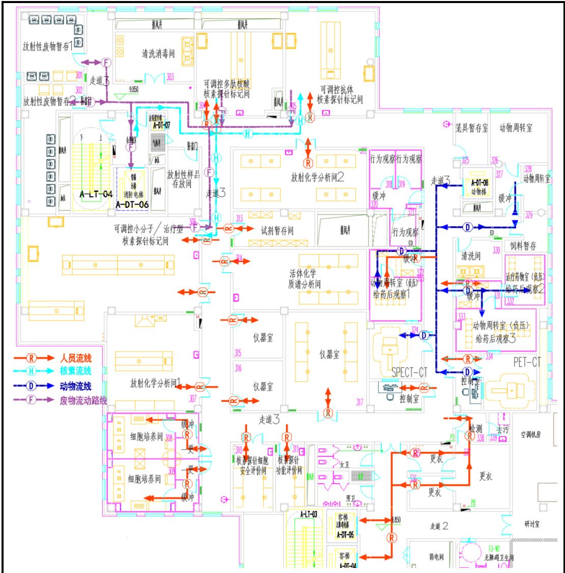
图 9-5 同位素实验室分区、人流物流和同位素路径示意图
